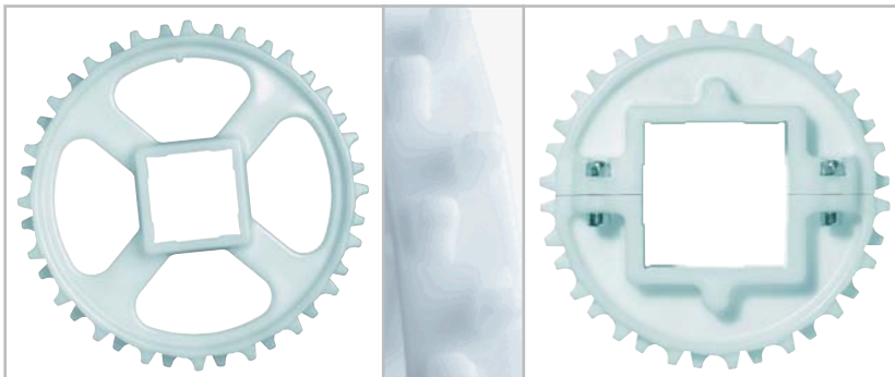
Неразборная звездочка с отверстиями (S)
